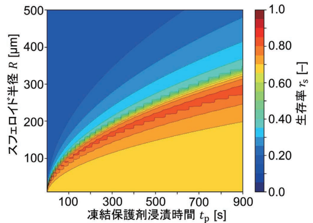
図3 生存率分布
