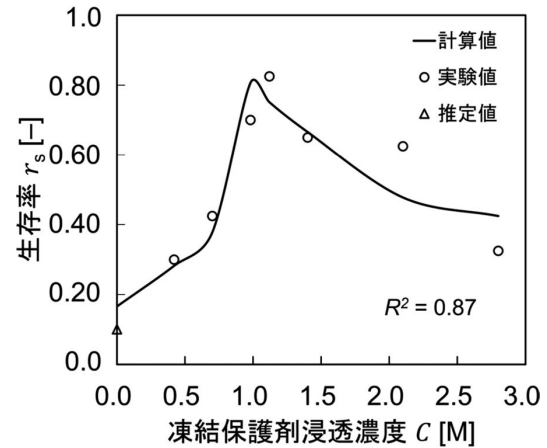
図2 生存率曲線
