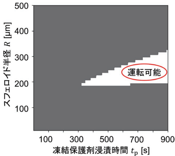
図4 凍結プロセスの運転可能領域
